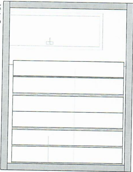
Vista C esc. 1/25
