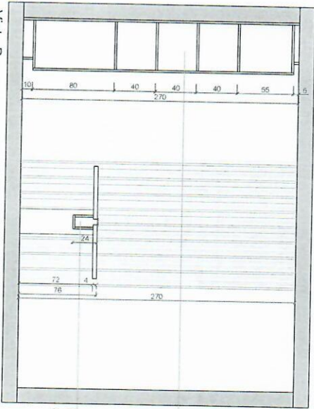
Planta baixa 01 esc. 1/25
